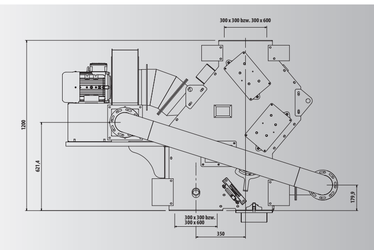
Schnitt | cross-section
